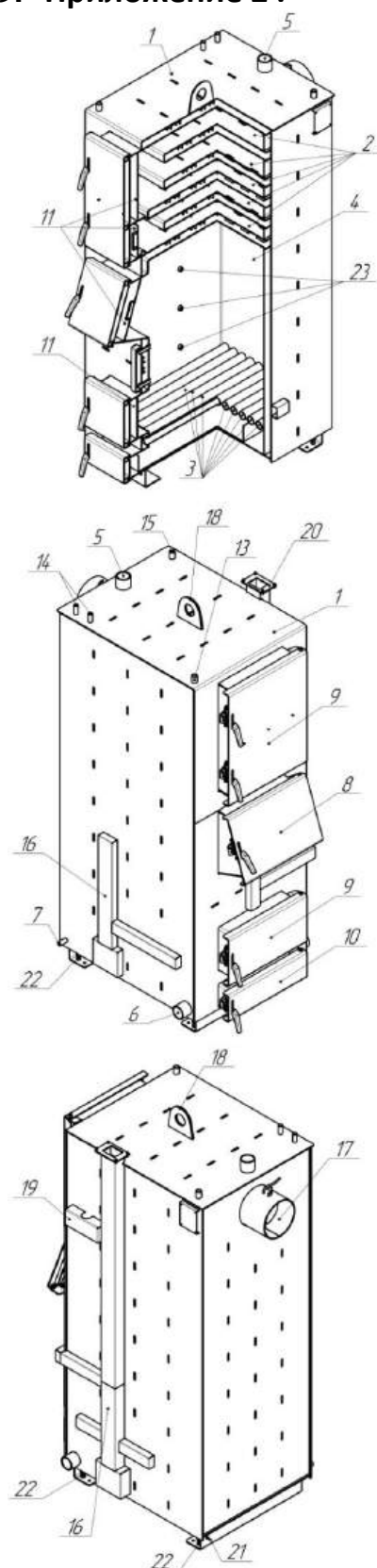
Рис. 6 Схема устройства отопительного кола HUNTEL «HOT 30», HUNTEL «HOT 40», HUNTEL «HOT 50», HUNTEL «HOT 60», HUNTEL «HOT 80», HUNTEL «HOT 110».
