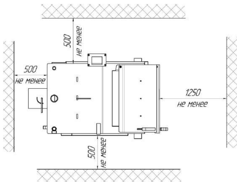
Рис. 1 Схема установки котла
