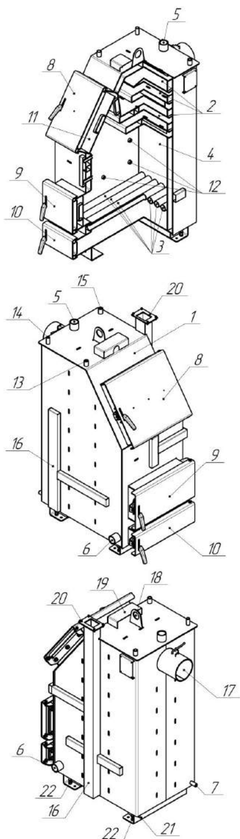
Рис. 5 Схема устройства отопительного кола HUNTEL «HOT 15», HUNTEL «HOT 20», HUNTEL «HOT 30».
